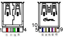
母头焊接面
